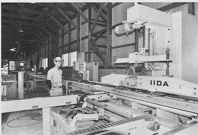
球磨杉の強度と含水率を測定し表示するグレーディングマシン
