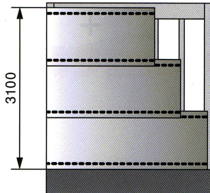
〈ジョシーツLX®11〉(重ね幅100ミリ)
